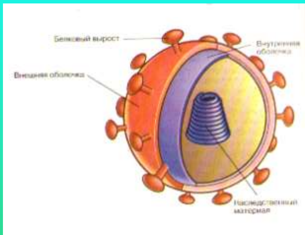
Схема строения вируса иммунодефицита человека (ВИЧ), увеличенного в 200 тыс. раз.
